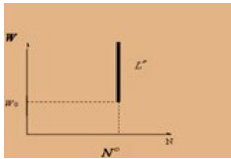
الشكل (1-3): منحنى عرض العمل
