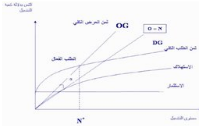
الشكل (1-1): منحني الطلب الفعال
