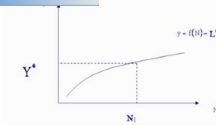
الشكل (1-2): منحنى الطلب على العمل
