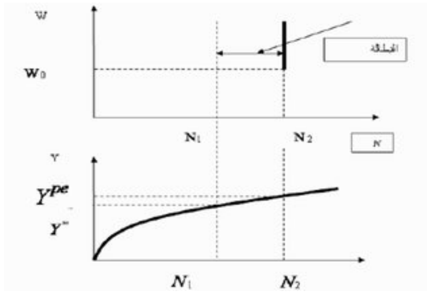
الشكل (1-4): منحنى يبين مستوى البطالة اللاإرادية
