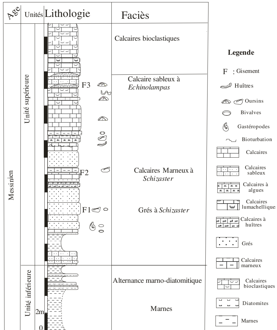
Fig. 09 : colonne lithologique de la coupe de sidi Abdelkader (Jdiouia)
