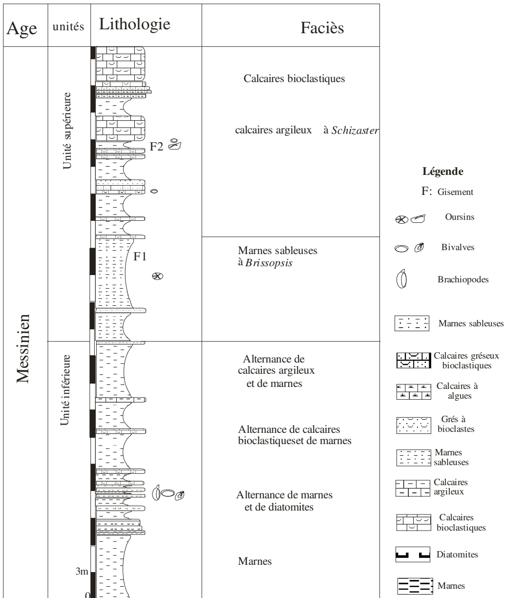
Fig. 08: colonne lithologique de la coupe de Jdiouia
