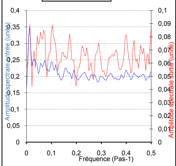
Amplitudes spectrales Troncature : 116 jours Pas : 1440 min Pas de calcul : 1 PK50-1987-88
