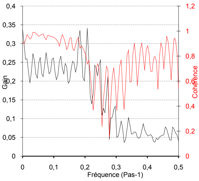
Amplitudes spectrales Troncature : 106 jours Pas : 1440 min Pas de calcul : 1 PK50-1984-1985
