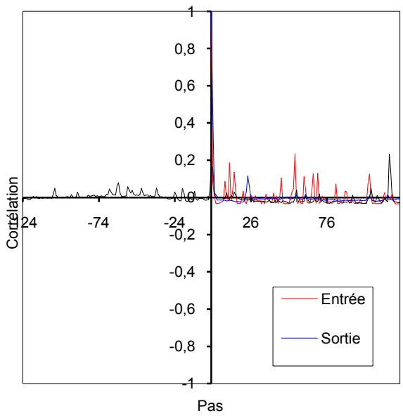
Corrélogrammes simples et croisés Troncature : 124 jours Pas : 1440 min Pas de calcul : 1 PK50-1992-93
