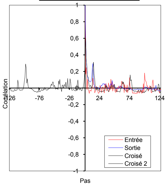
Corrélogrammes simples et croisés Troncature : 126 jours Pas : 1440 min Pas de calcul : 1 PK50-1991-92
