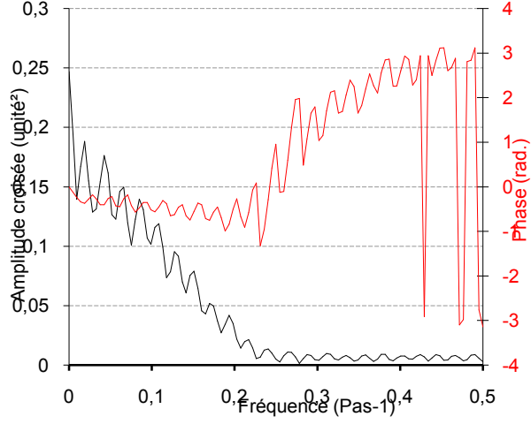
Fonctions d'amplitude croisée et de phase Troncature : 106 jours Pas : 1440 min Pas de calcul : 1 PK50-1984-1985
