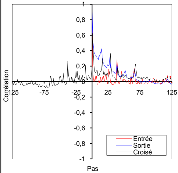
Corrélogrammes simples et croisés Troncature : 125 jours Pas : 1440 min Pas de calcul : 1 pk50-82-83
