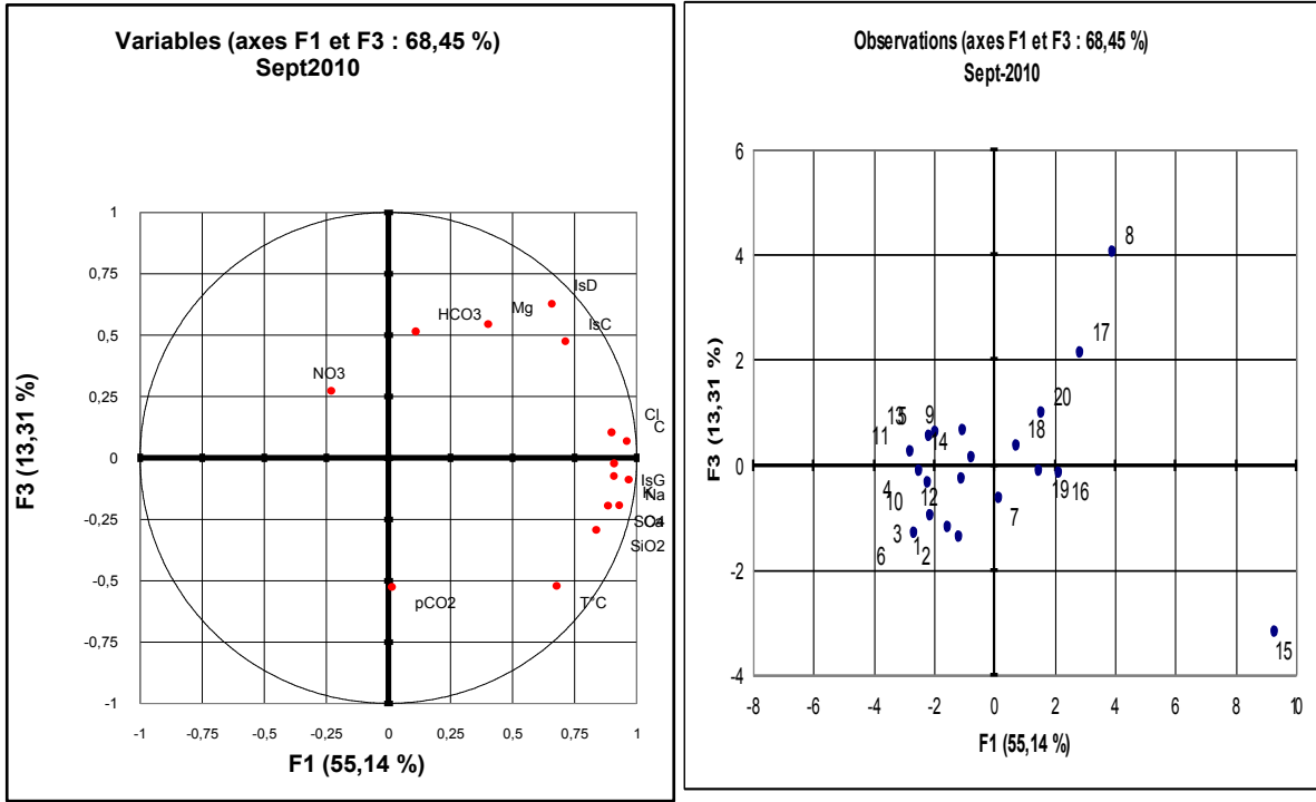
Figure 96: ACP de la campagne de septembre 2010 Plan principal F1-F3 des variables (à gauche) et des échantillons (à droite).
