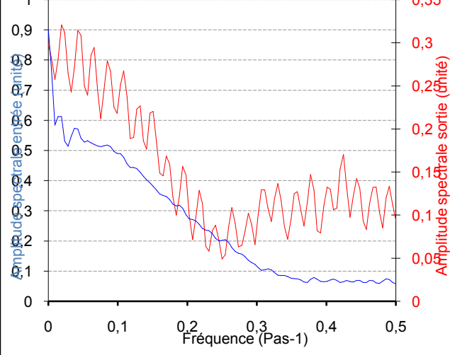
Amplitudes spectrales Troncature : 106 jours Pas : 1440 min Pas de calcul : 1 PK50-1984-1985
