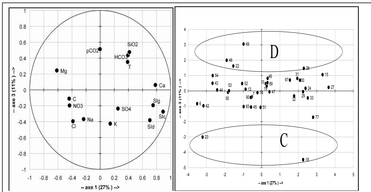
Figure 82: ACP de la campagne de mai 1992 pour les forages. Plan principal F1-F3 des variables (à gauche) et des échantillons (à droite).
