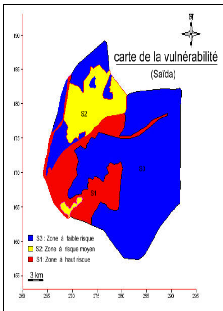
Figure 102: Carte de vulnérabilité de la zone d'alimentation de l'aquifère karstique de Saïda.
