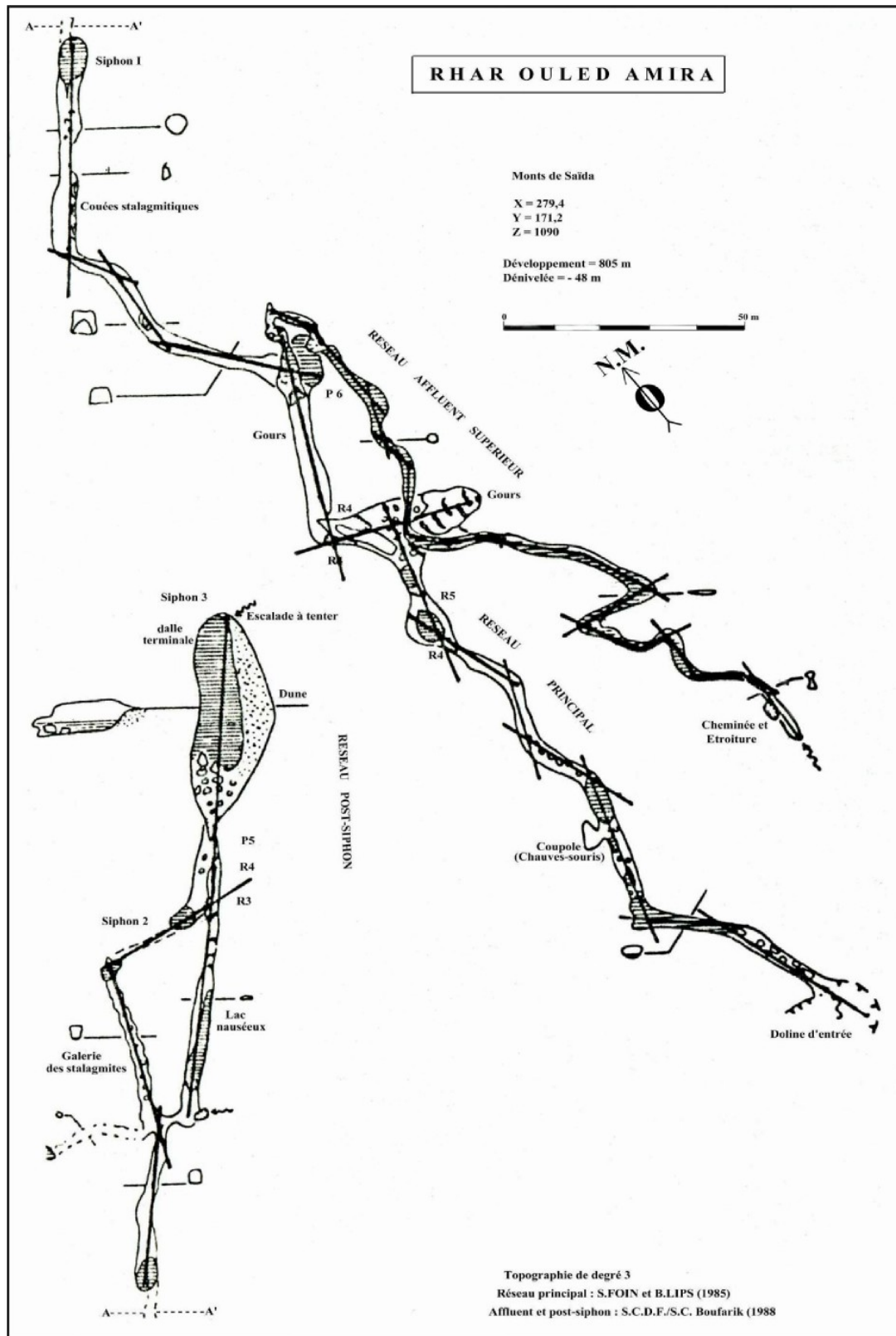
Figure 31: Schéma de configuration de la perte de Rhar O. Amira (S.Foin et B.Lips,1985).
