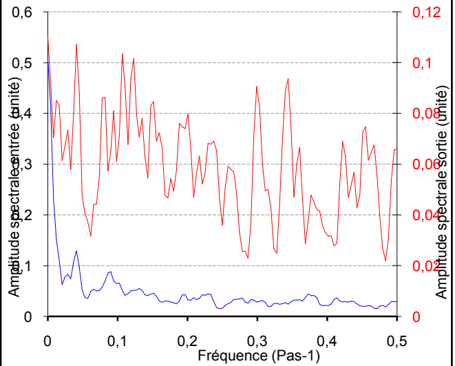
Amplitudes spectrales Troncature : 122 jours Pas : 1440 min Pas de calcul : 1 PK50-1983-84
