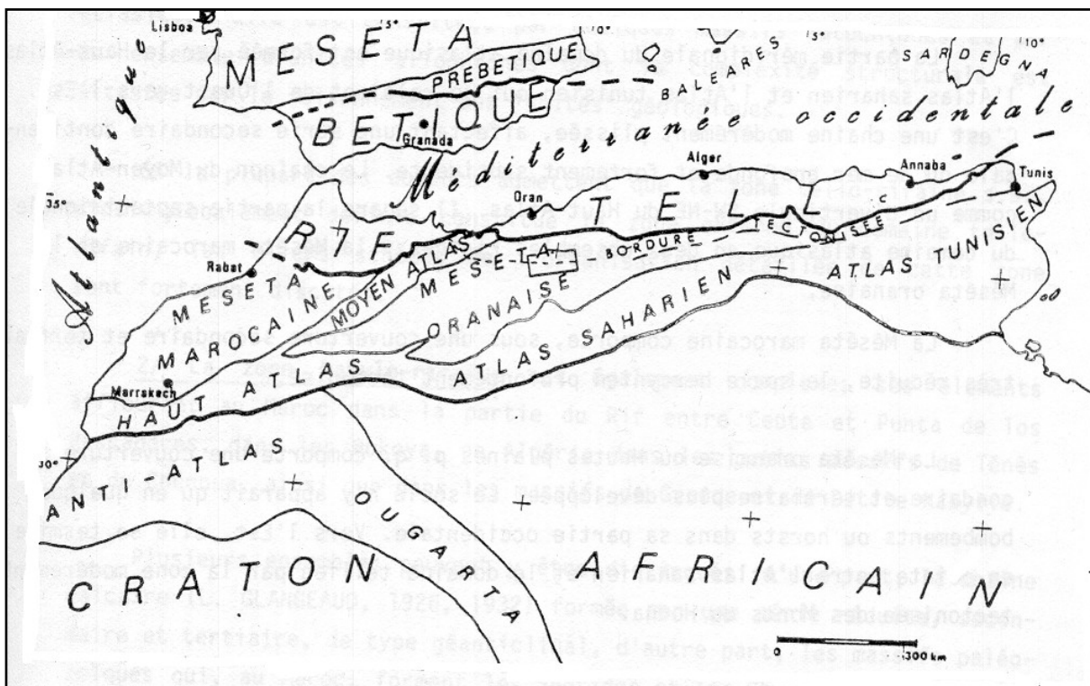
Figure1: Extrait de la carte géologique d'Algérie (Guardia ,1975).
