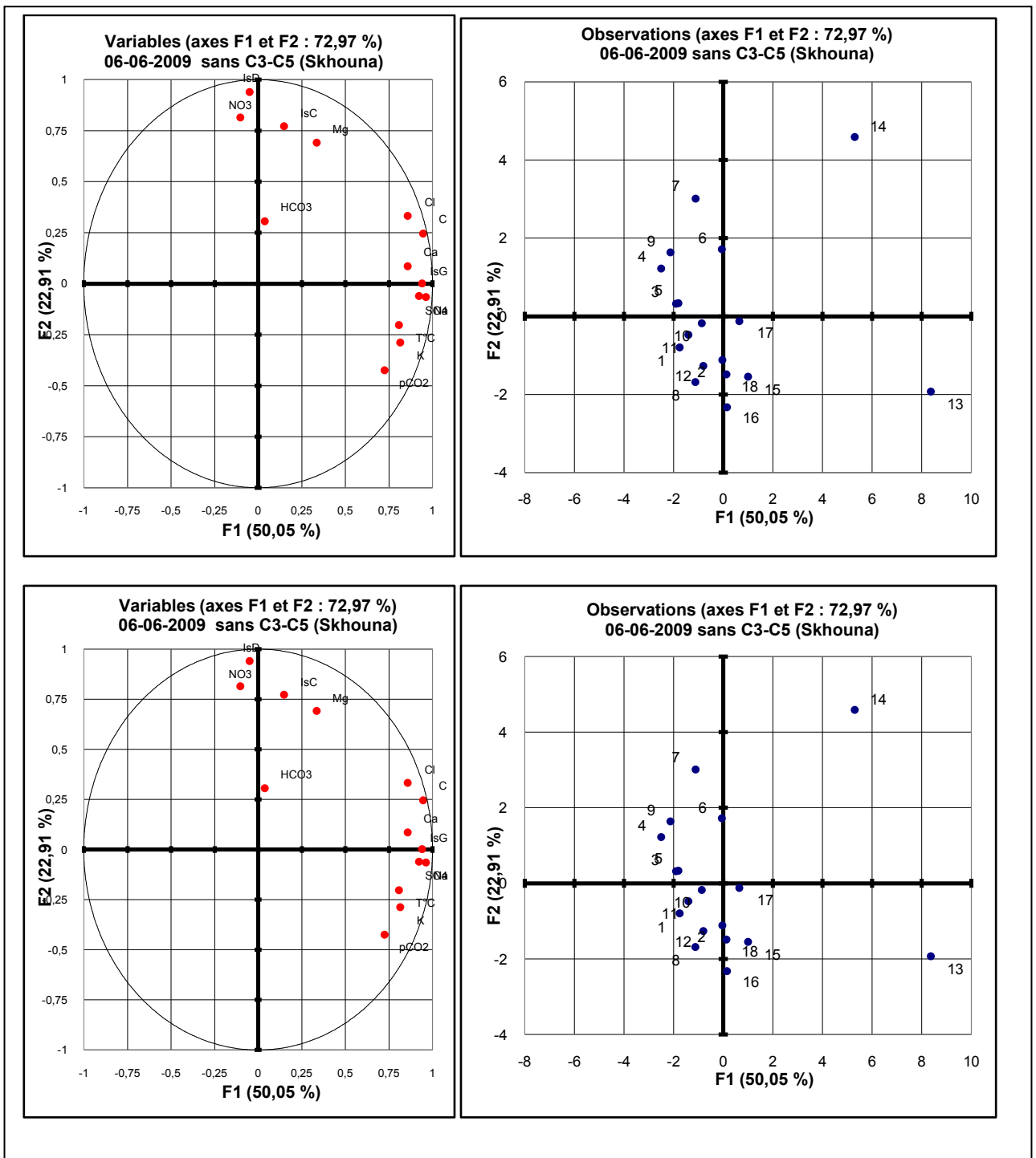
Figure : ACP de Juin 2009 (sans C3etC5) Plan des variables (à gauche) échantillons (à droite).3:ELBorj . 4 :Benadouene ; 5:A,Sultane ; 7 :F1 ; 8 :FIITGC .; 6 :A.Zerga ; 9:S.Embarek; 8 :P/Zerouki ;10:F/Tamesna 11: F/Tifrit ;12: Sidi Gacem; 13:F62;14: F4; 15: F27 ; 16 : P/Hamam Rabi; 17 : F1-Youb ; 18 : F/Hassi ElAbd; 19 :F/Maata ; 20:F2-Youb; 21: F/Bouriche.
