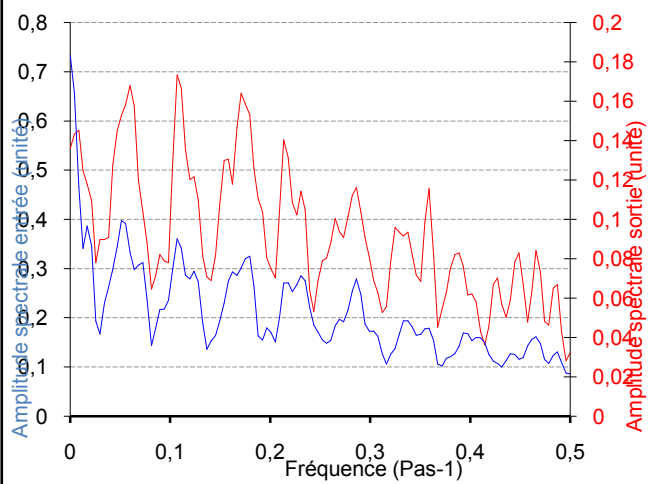
Amplitudes spectrales Troncature : 117 jours Pas : 1440 min Pas de calcul : 1 PK50-1987-88
