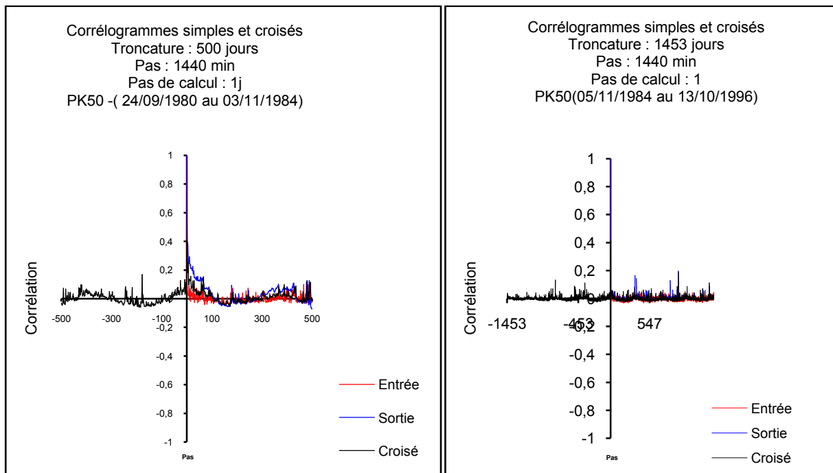
Figure 61: Corrélogrammes croisés du PK50 -Périodes de 1980-84 et 1984-96.
