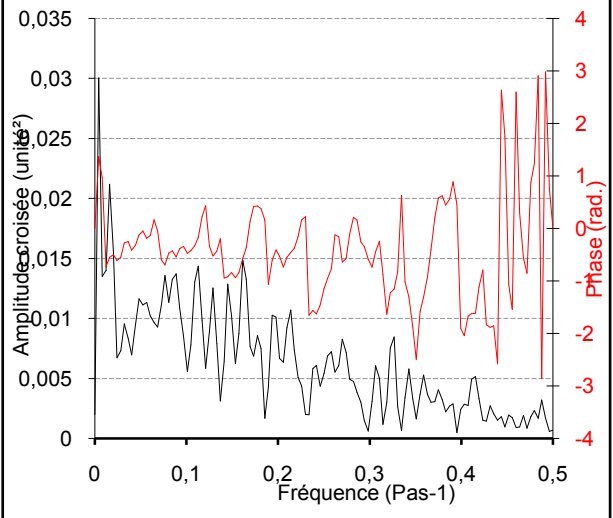
Fonctions d'amplitude croisée et de phase Troncature : 124 jours Pas : 1440 min Pas de calcul : 1 PK50-1992-93
