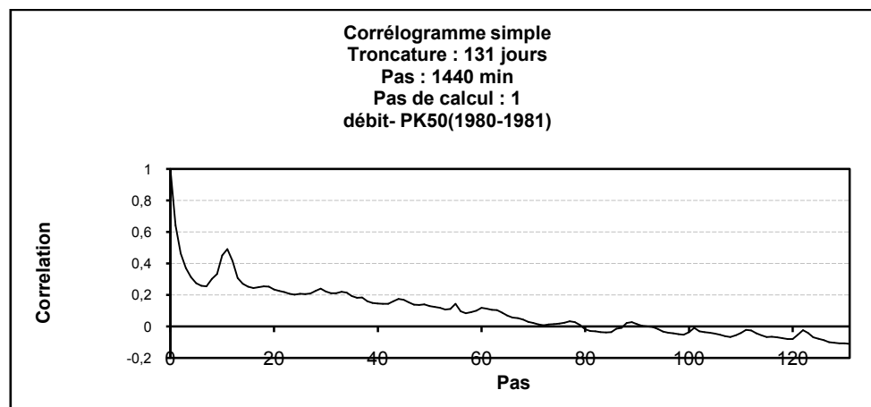
Figure 53: Corrélogramme simple des débits à la station du PK50 -cycle 1980-1981.
