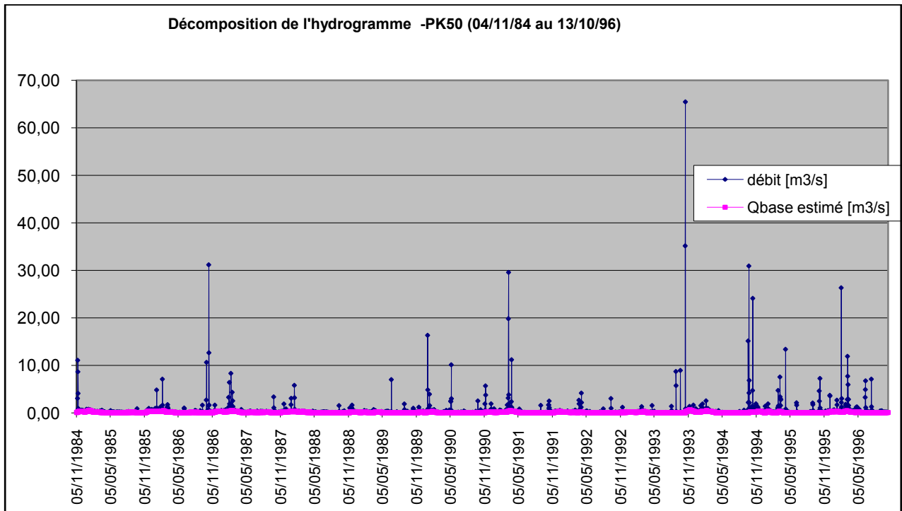
Figure 51: Décomposition de l'hydrogramme à la station PK 50 Période du 05/11/1984 au 13/10/1996.
