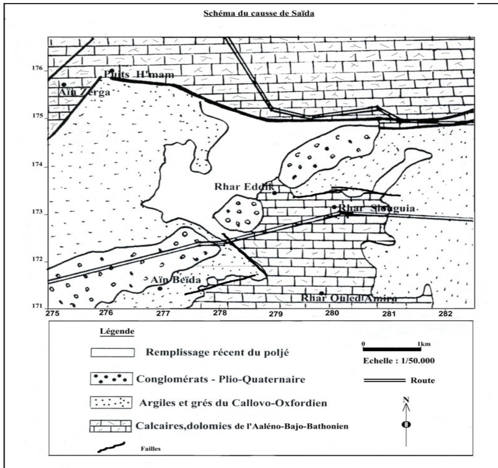
Figure 26: Schéma du causse de Saïda.
