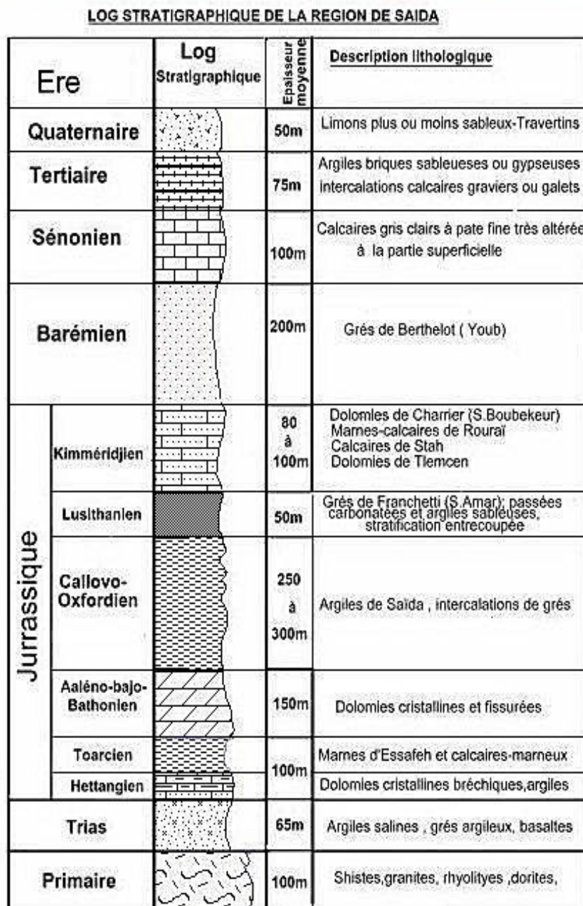
Figure 6 : Log stratigraphique de la région de Saïda.
