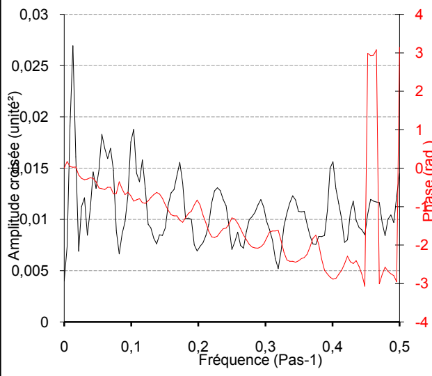
Fonctions d'amplitude croisée et de phase Troncature : 116 jours Pas : 1440 min Pas de calcul : 1 PK50-1988-89
