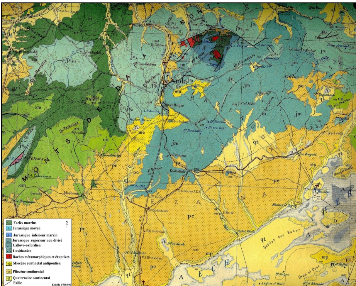
Figure 5 : Carte géologique de la région de Saïda
