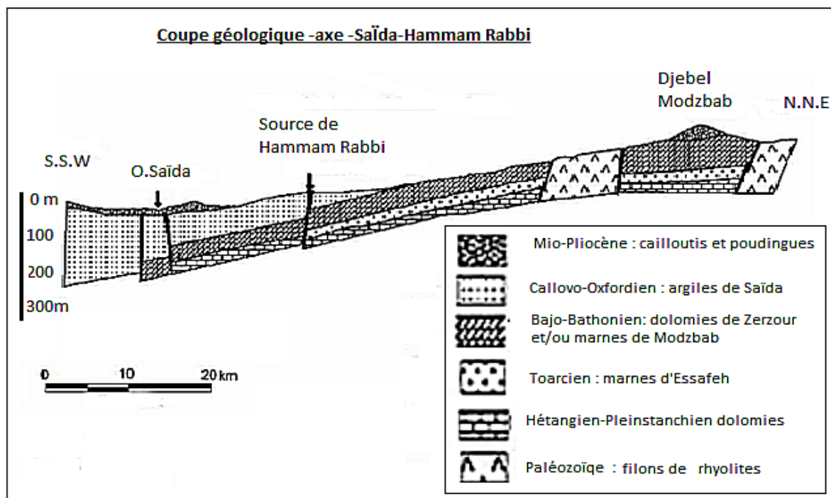
Figure 12: Coupe géologique axe Saïda-Hammam Rabbi( Etude SATEC,1995).
