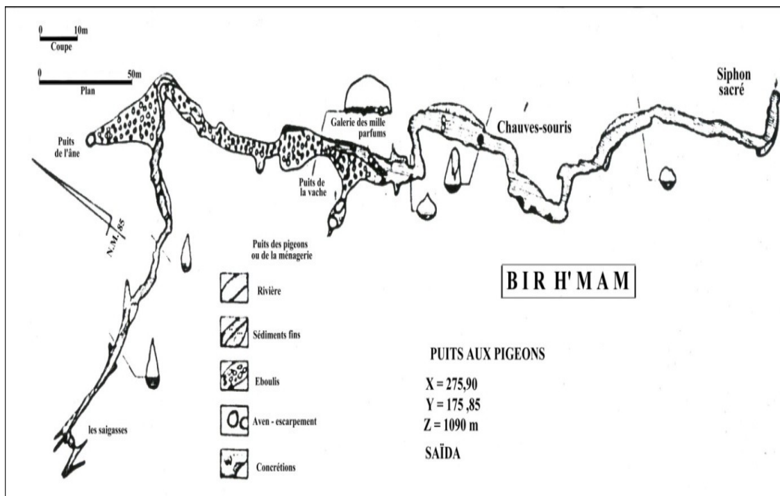
Figure 30 : Schéma de la perte de Bir H'mam (S.Foin et B.Lips,1985).
