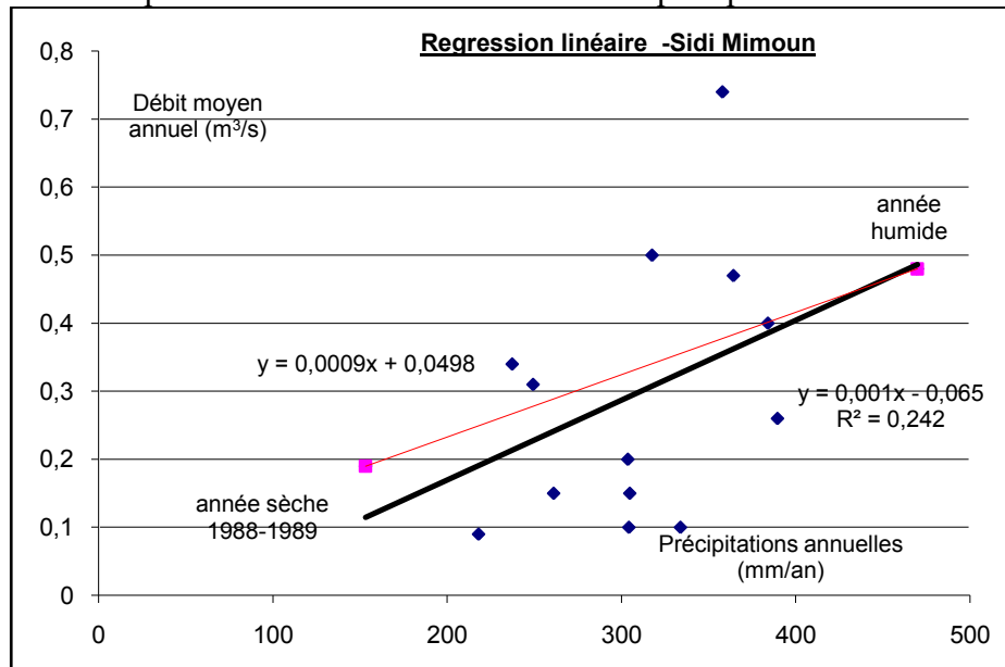
Figure 25: Droite de régression linéaire (Pluie-Débit)-Sidi Mimoun.
