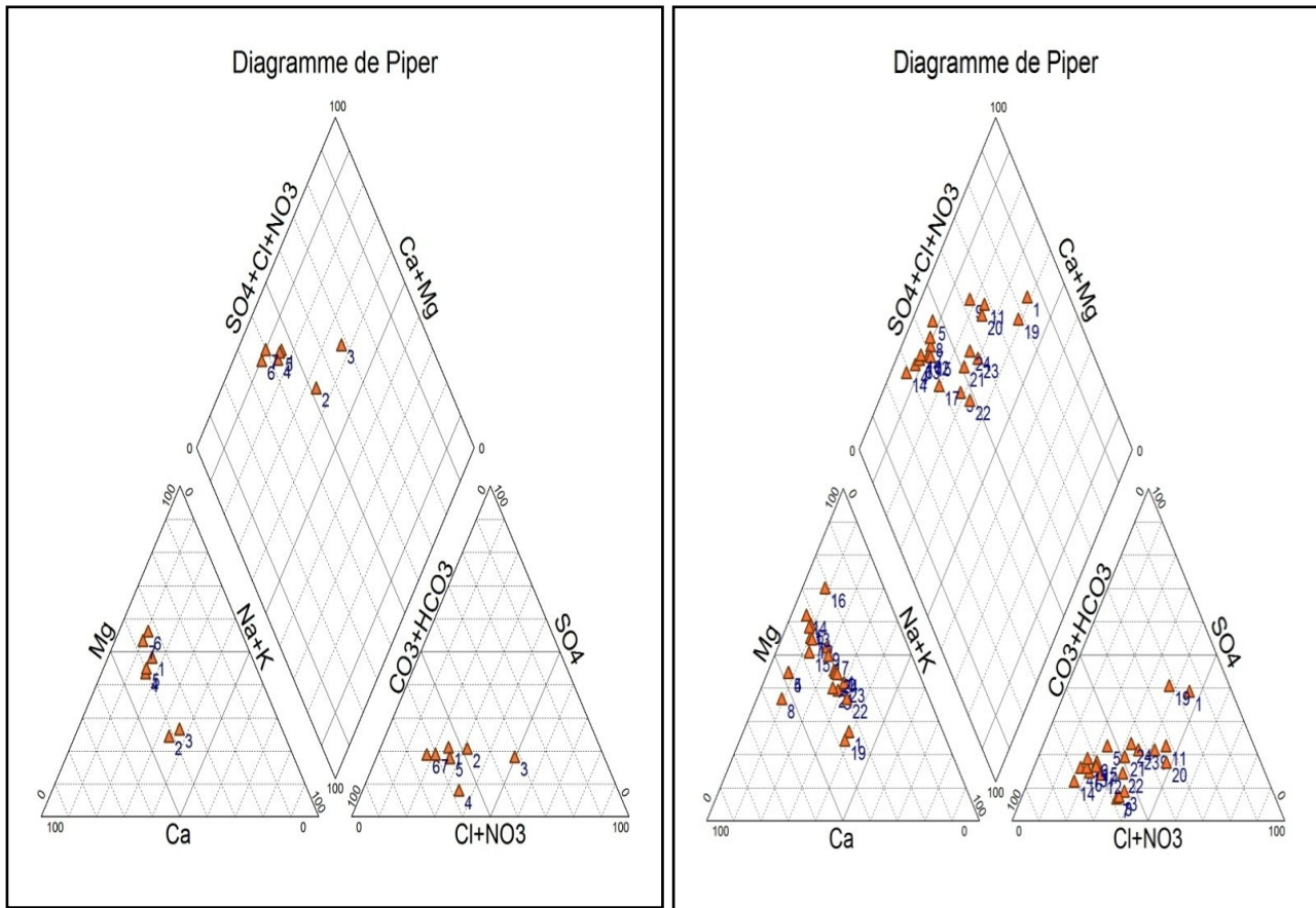
Figure 91: Diagrammes de Piper des points analysées (à gauche sources -avril 2010-), (à droite les forages et sources -septembre 2010).
