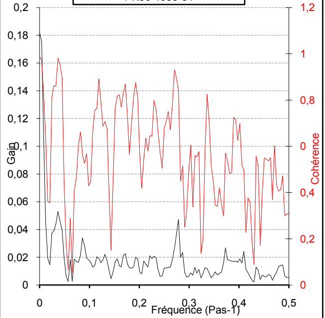
Fonctions de gain et de cohérence Troncature : 122 jours Pas : 1440 min Pas de calcul : 1 PK50-1983-84
