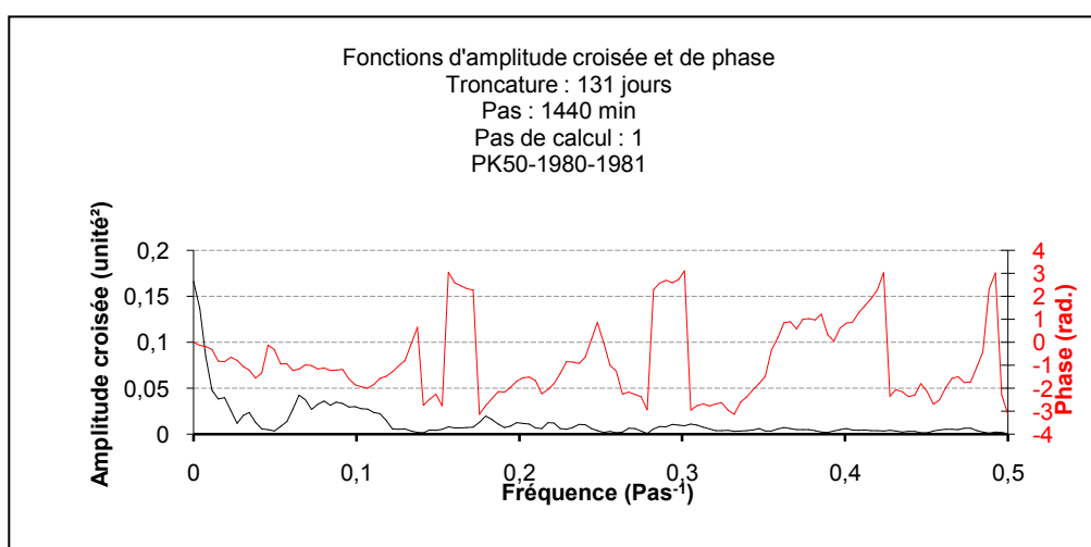
Figure 55: Amplitude croisée et phase PK50 -cycle 1980-1981.
