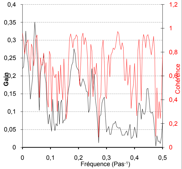
Fonctions de gain et de cohérence Troncature : 125 jours Pas : 1440 min Pas de calcul : 1 PK50-81-82
