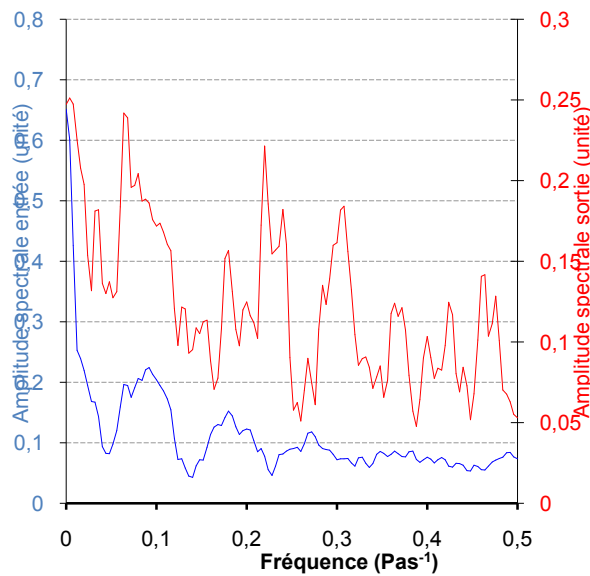
Amplitudes spectrales Troncature : 125 jours Pas : 1440 min Pas de calcul : 1 PK50-80-81
