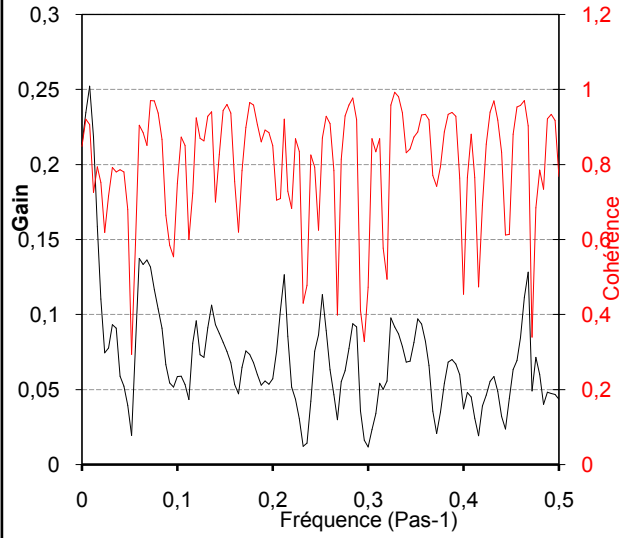
Fonctions de gain et de cohérence Troncature : 125 jours Pas : 1440 min Pas de calcul : 1 PK50-82-83
