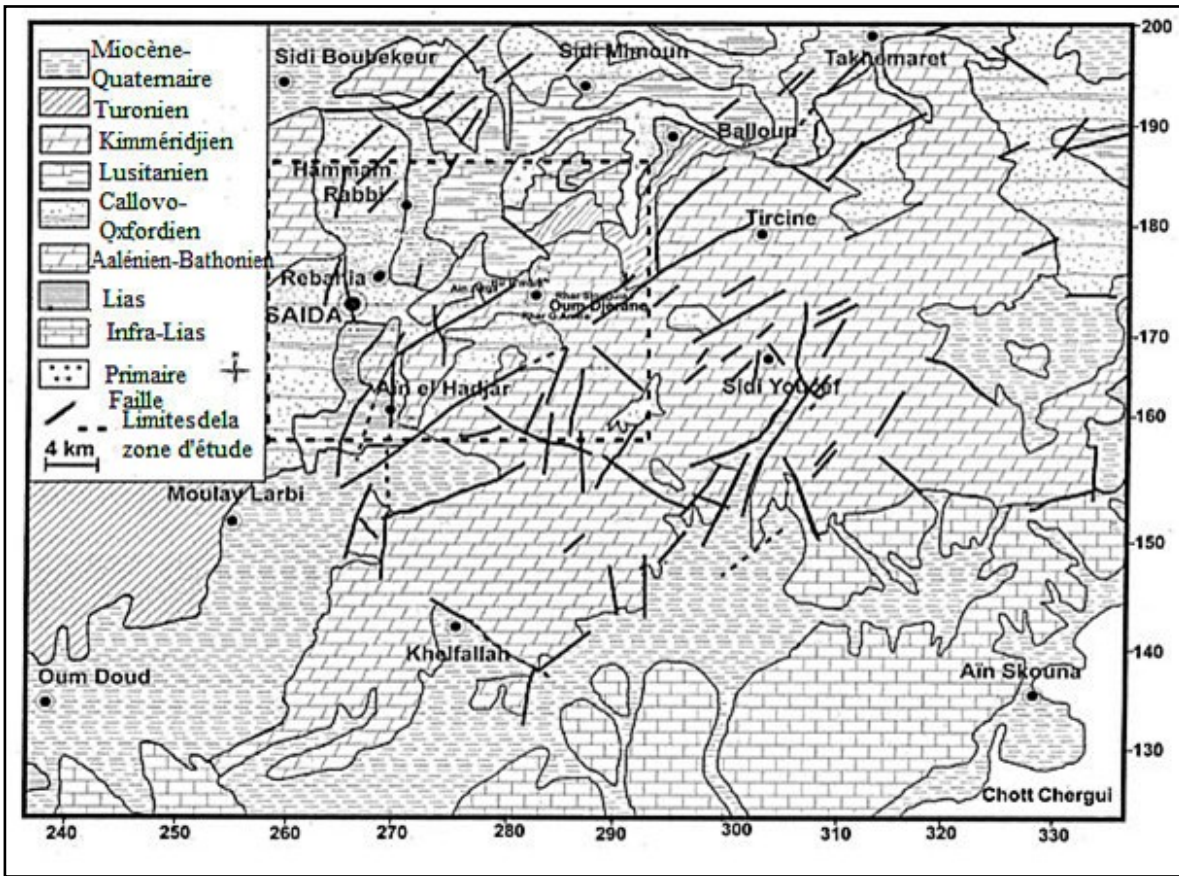
Figure 7: Lithologie et tectonique de la zone d'étude.
