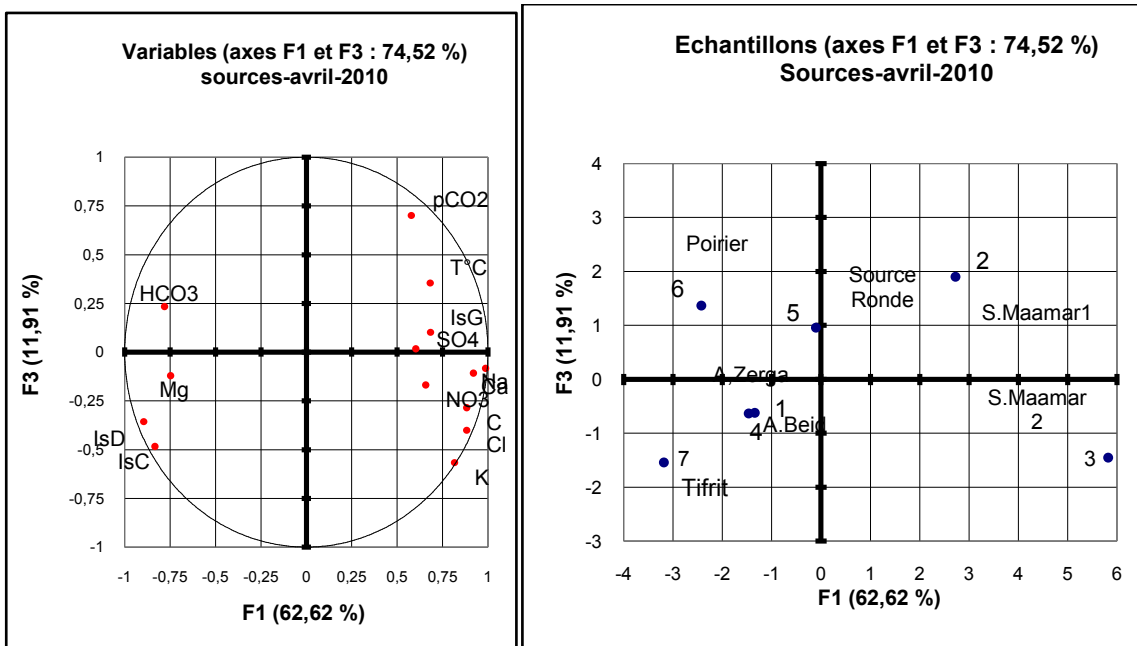
Figure94: ACP de la campagne d'avril 2010 Plan principal F1-F3 des variables (à gauche) et des échantillons (à droite).
