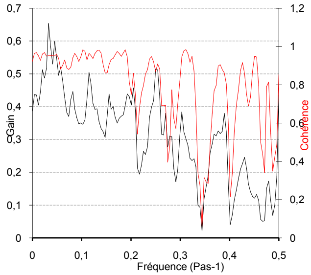
Amplitudes spectrales Troncature : 122 jours Pas : 1440 min Pas de calcul : 1 PK50 (1990-91)
