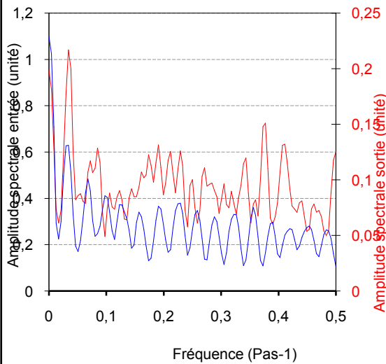
Amplitudes spectrales Troncature : 118 jours Pas : 1440 min Pas de calcul : 1 PK50-1985-86
