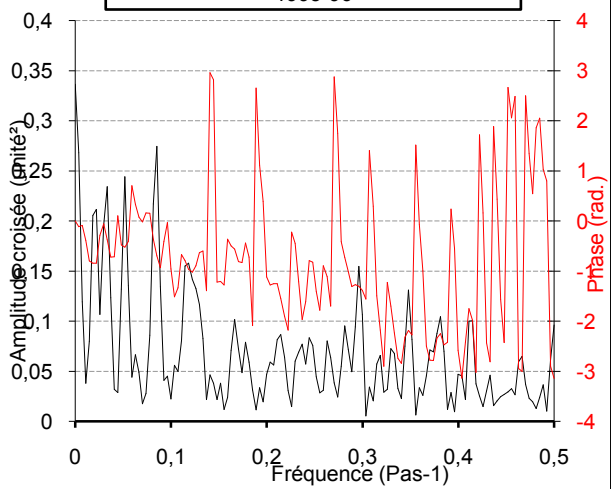
Fonctions d'amplitude croisée et de phase Troncature : 135 jours Pas : 1440 min Pas de calcul : 1 1995-96
