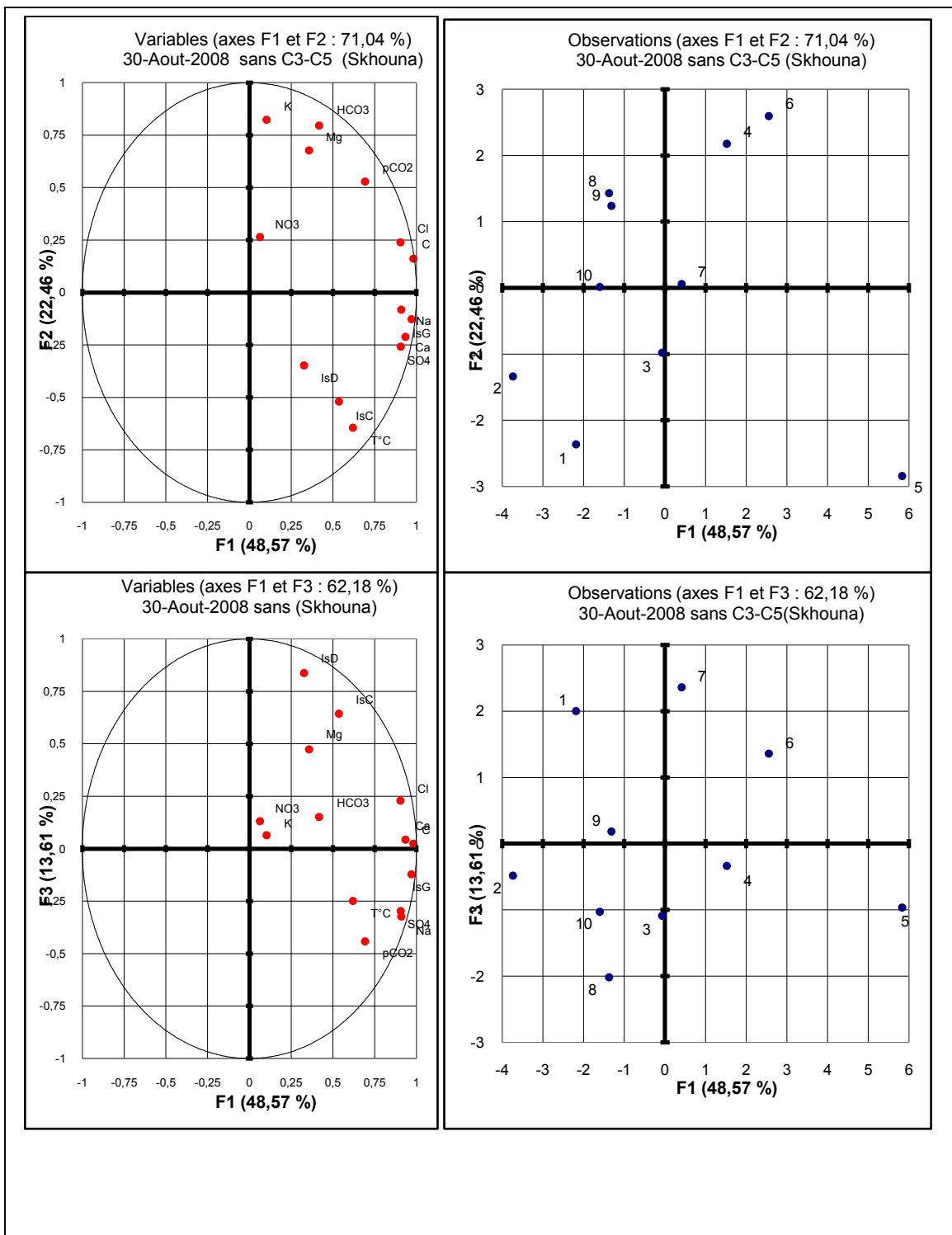
Figure : ACP d'Aout2008 Plan des variables (à gauche) échantillons (à droite).
