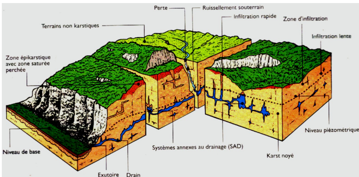
Figure32 : Représentation d'un système karstique (d'après A.Mangin in Groundwater Ecology, 1994).
