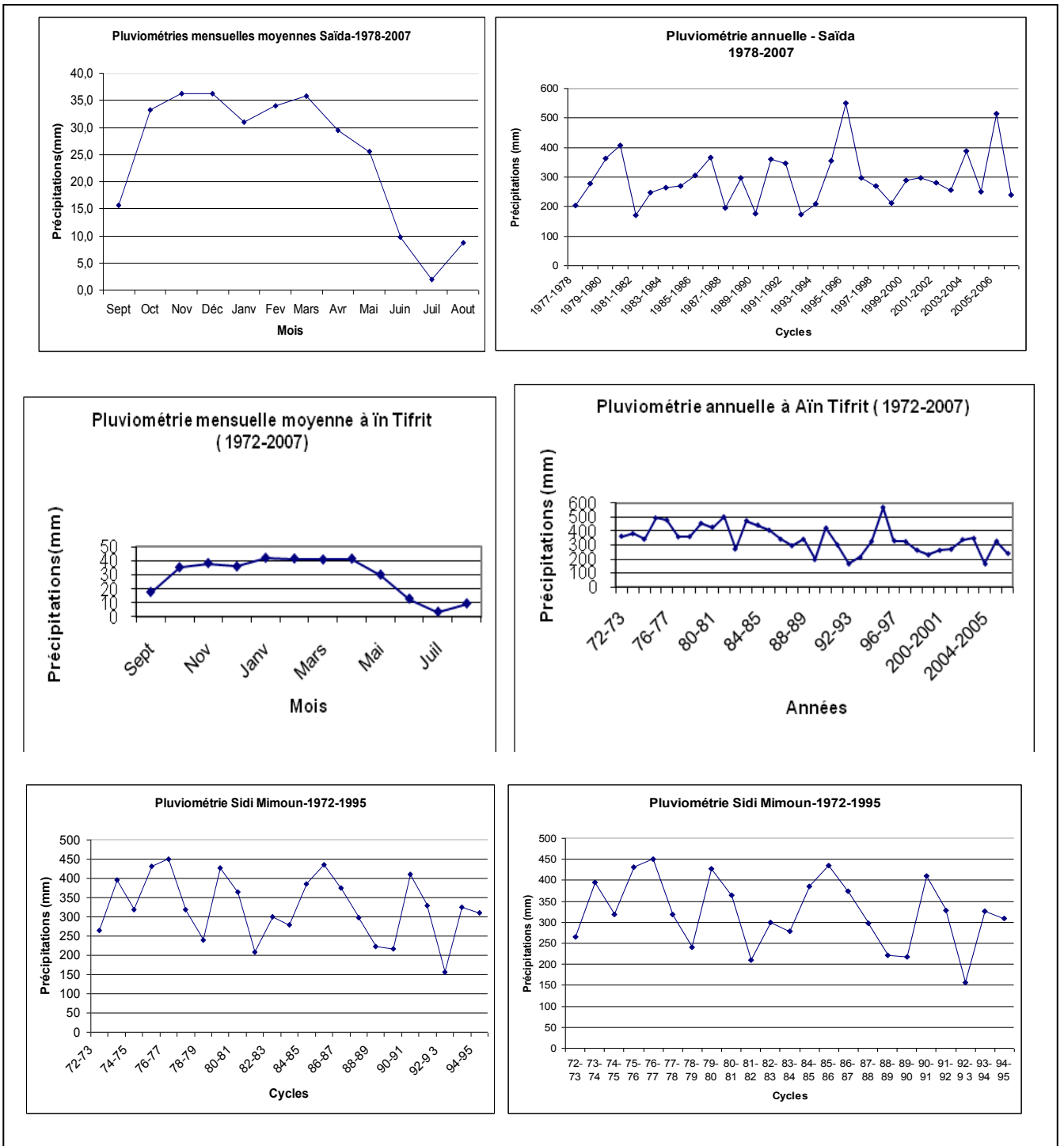
Figure 18: Pluviométries mensuelles et annuelles enregistrées au niveau des stations de Saïda, Tifrit et S.Mimoun.
