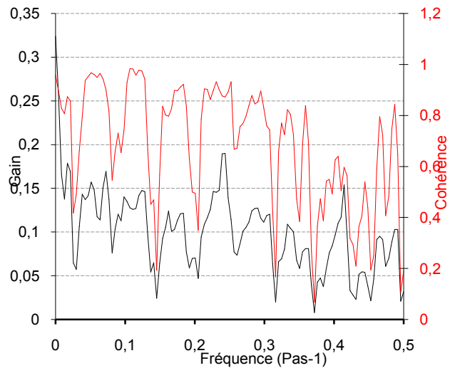
Amplitudes spectrales Troncature : 117 jours Pas : 1440 min Pas de calcul : 1 PK50-1987-88
