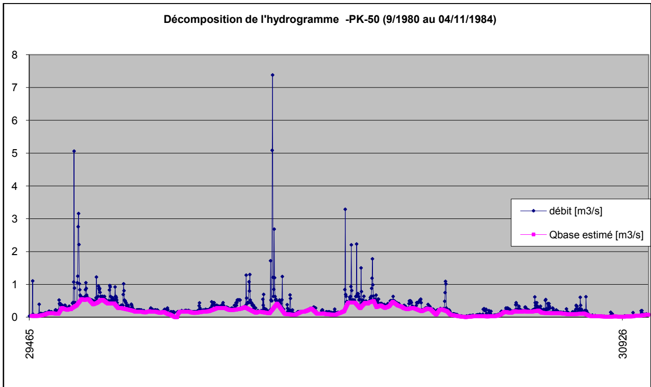
Figure 50 : Décomposition de l'hydrogramme à la station PK 50 Période du 01/09/1980 au 04/11/1984
