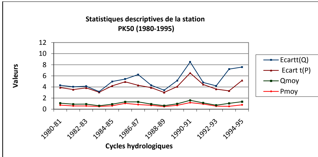
Figure 20 : Statistiques descriptives de la station du PK50.
