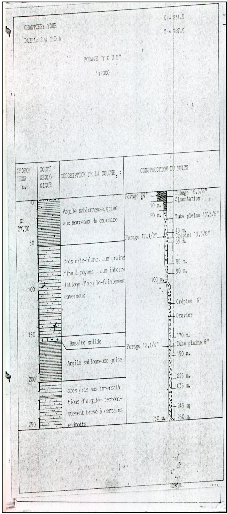
Figure. : Coupe géologique du forage de YOUB.
