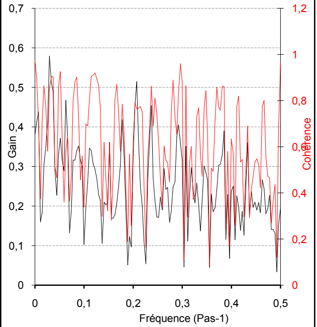
Amplitudes spectrales Troncature : 135 jours Pas : 1440 min Pas de calcul : 1 1995-96
