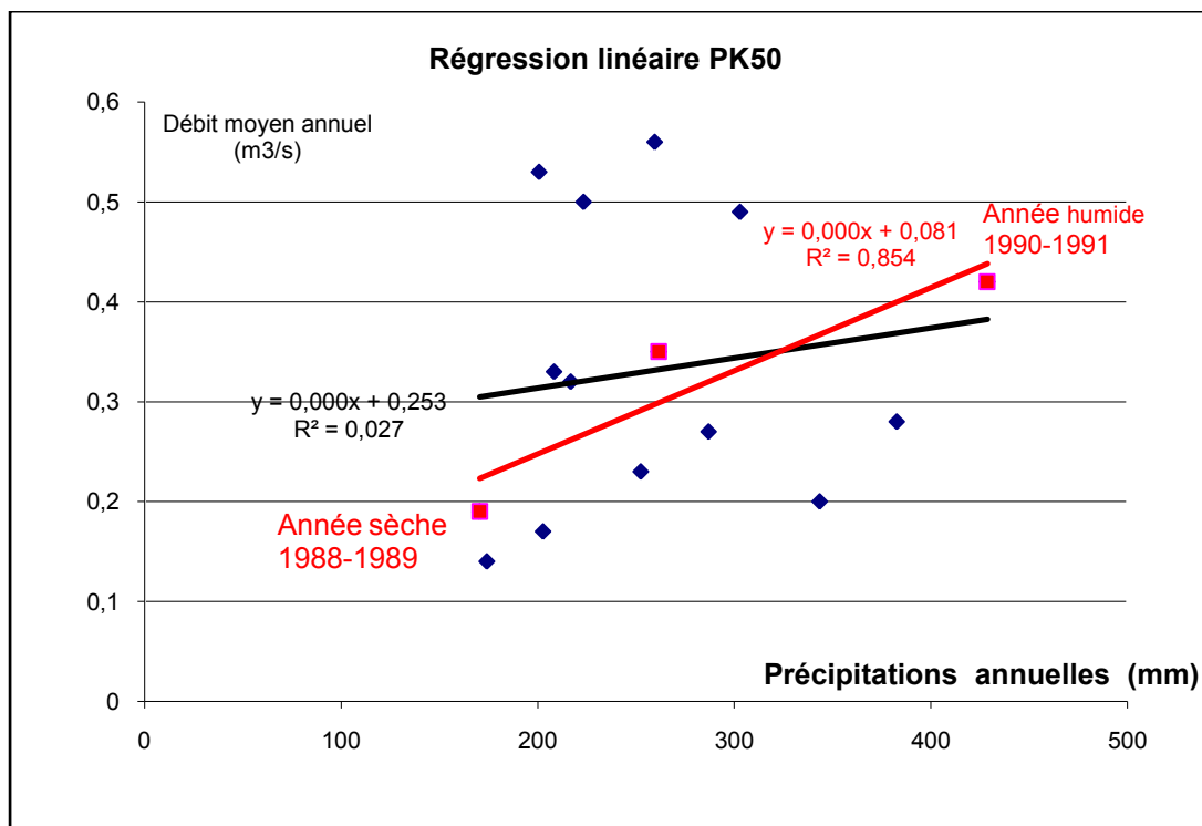
Figure 24: Droite de régression linéaire (Pluie-Débit) PK50-(1980-1995).
