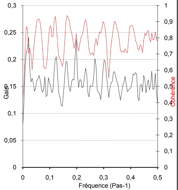
Fonctions de gain et de cohérence Troncature : 116 jours Pas : 1440 min Pas de calcul : 1 1988-89
