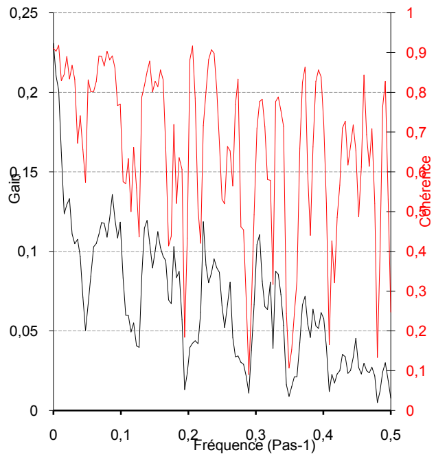
Fonctions de Gain et Coherence Troncature: 126 jour Pas: 1440 Pas de calcul : 1 PK50-1991-1992
