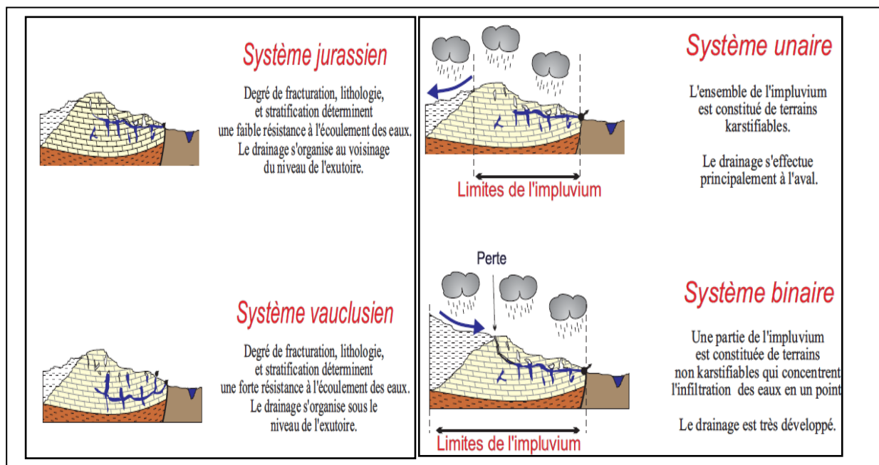
Figure 33 : Les différentes configurations des karsts (Marsaud, 1996).
