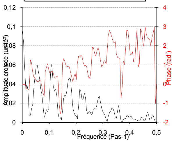
Fonctions d'amplitude croisée et de phase Troncature : 117 jours Pas : 1440 min Pas de calcul : 1 PK50-1987-88
