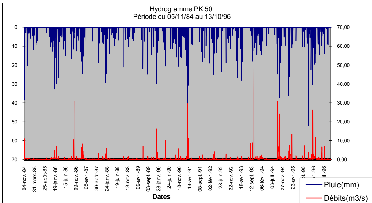
Figure 59 : Hydrogramme du PK50 -Période du 05/11/84 au 13/10 /96.
