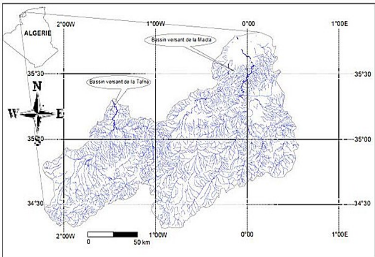
Figure 14: Réseau hydrographique de la région ouest (ANRH).
