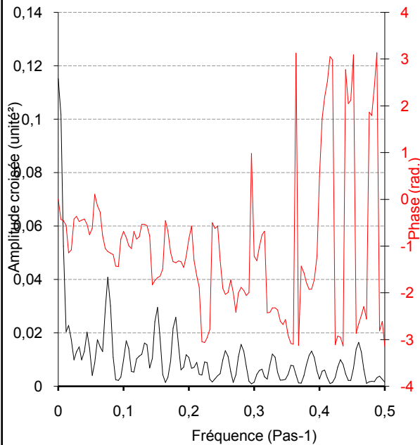
Fonctions d'amplitude croisée et de phase Troncature : 125 jours Pas : 1440 min Pas de calcul : 1 PK50-82-83
