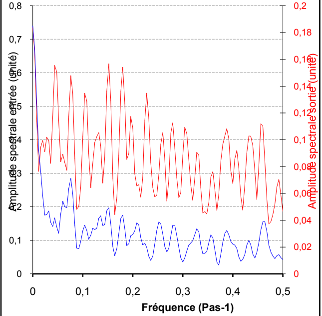
Amplitudes spectrales Troncature : 125 jours Pas : 1440 min Pas de calcul : 1 pk50-82-83
