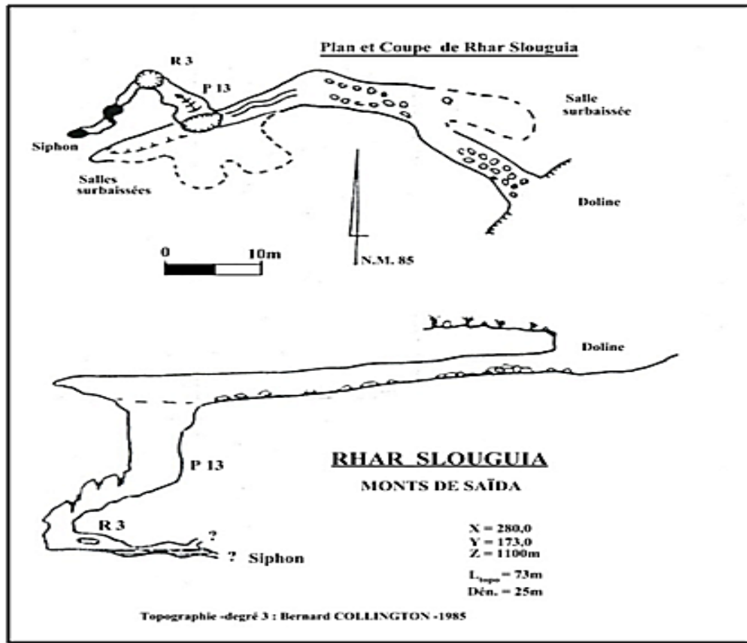
Figure 29 : Coupe et plan de la perte de Rhar Slougua (S.Foin et B.Lips,1985).
