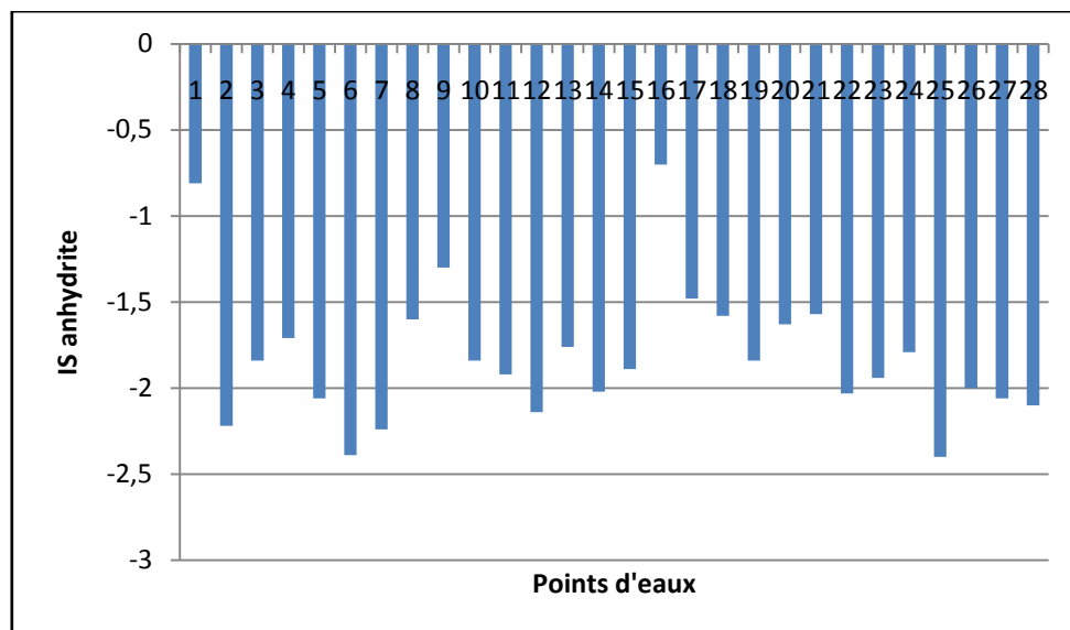
Figure 91: Indices de saturation de l'anhydrite dans les eaux des forages (1-21) et dans les sources (22-28).
