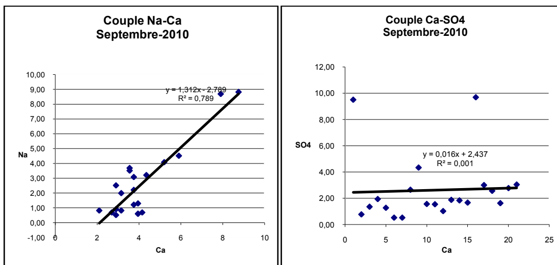
Figurexxx: Corrélation Ca-Na et Ca - SO4.
