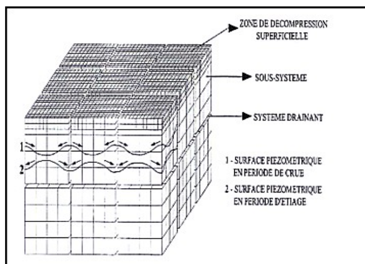
Figure 35 : Schématisation d'un système karstique (Drogue, 1971).
