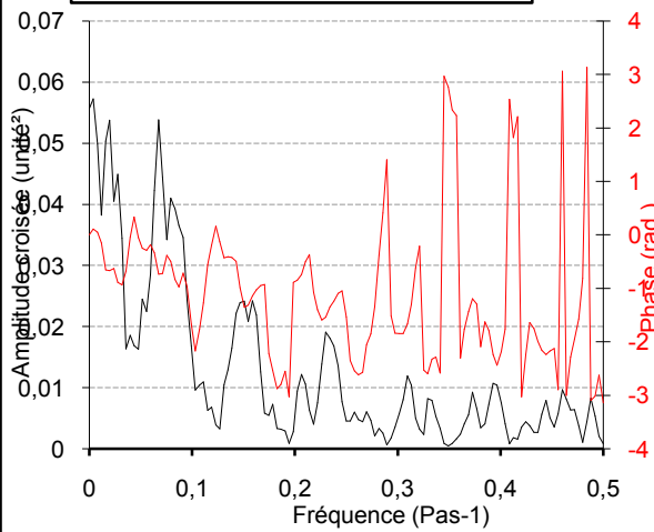
Fonctions d'amplitude croisée et de phase Troncature : 126 jours Pas : 1440 min Pas de calcul : 1 PK50-1991-1992
