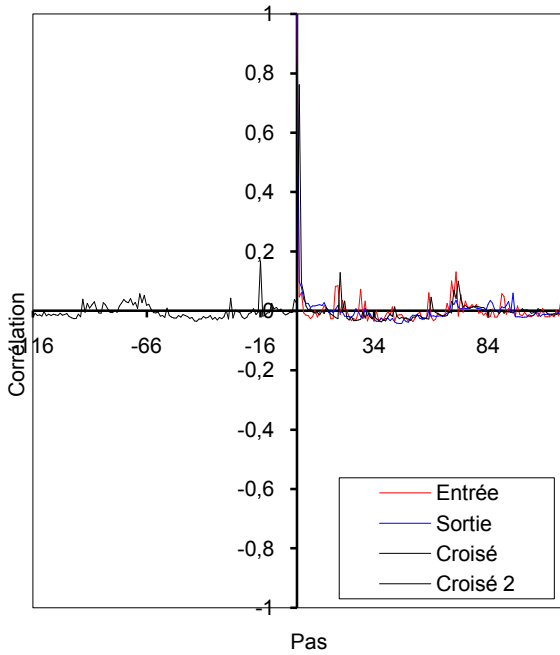
Corrélogrammes simples et croisés Troncature : 116 jours Pas : 1440 min Pas de calcul : 1 PK50-1988-89
