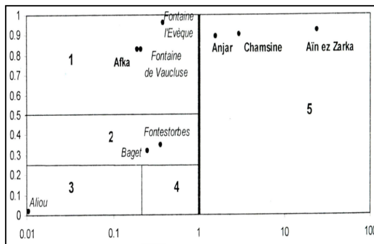
Figure 73: Classification des systèmes karstiques (Hakim, 2005).
