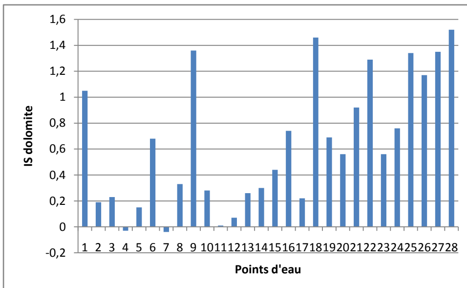
Figure 87: Indices de saturation de la dolomite dans les eaux des forages (1-21) et dans les sources (22-28)
