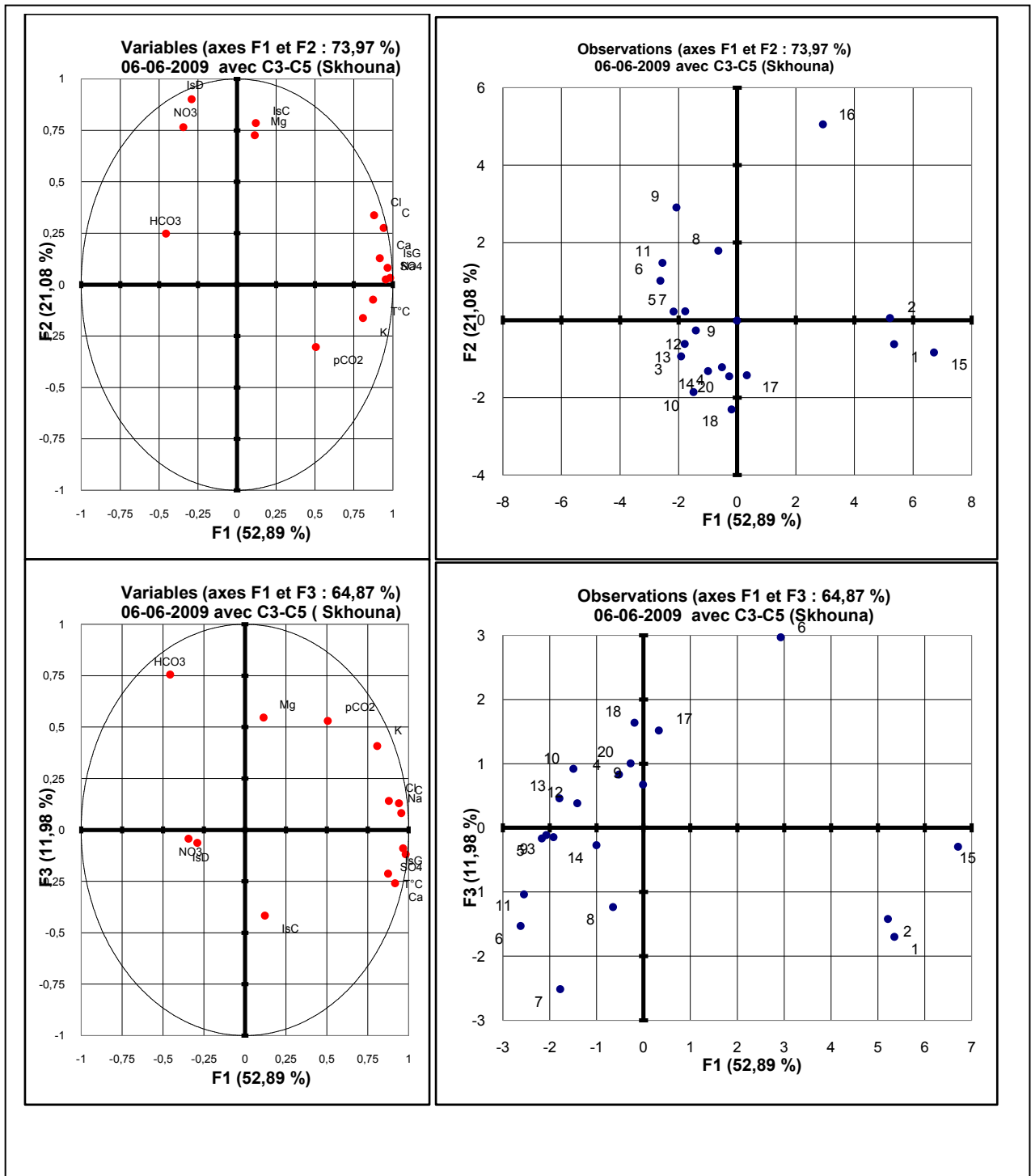
Figure : ACP de Juin 2009 (avec C3 et C5) Plan des variables (à gauche) échantillons (à droite).
