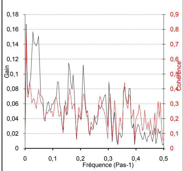
Fonctions de gain et de cohérence Troncature : 124 jours Pas : 1440 min Pas de calcul : 1j PK50(1992-93)
