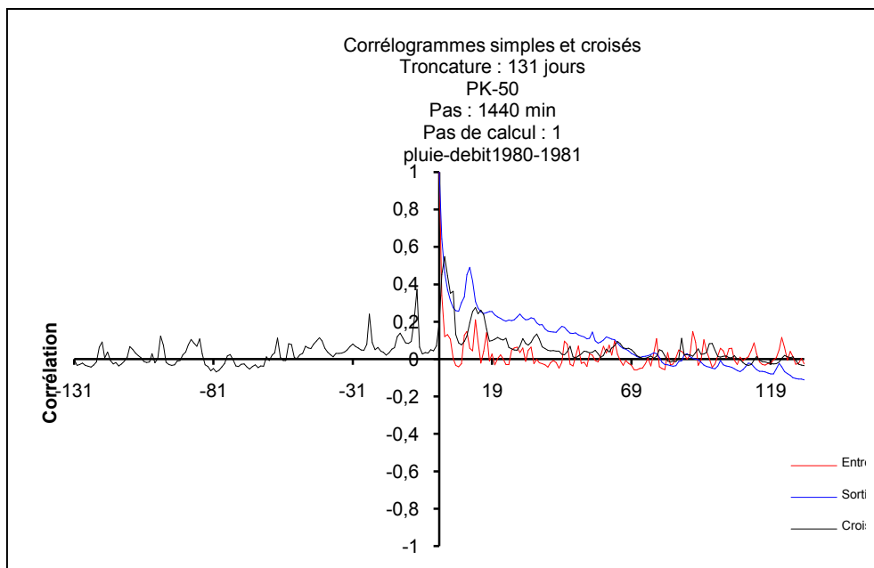
Figure 54: Corrélogramme croisé du PK50 -cycle 1980-1981.
