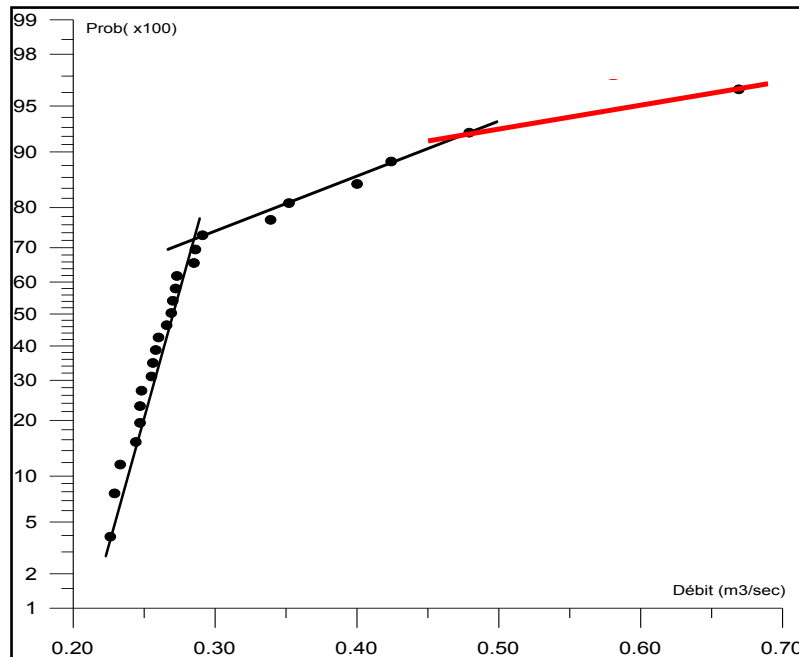
Figure 44 : Graphique des débits classés à Saïda.
