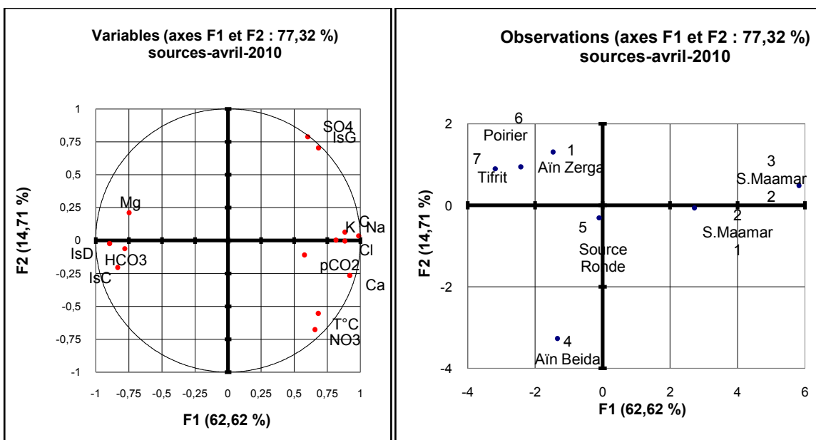
Figure93 : ACP de la campagne d'avril 2010 Plan principal F1-F2 des variables (à gauche) et des échantillons (à droite).
