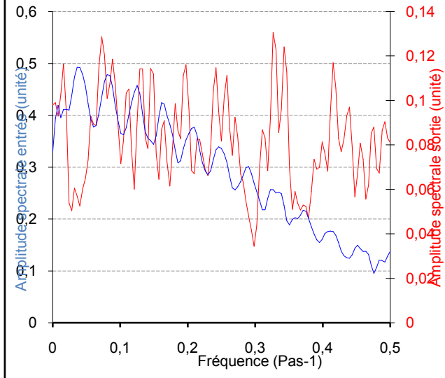
Amplitudes spectrales Troncature : 124 jours Pas : 1440 min Pas de calcul : 1
