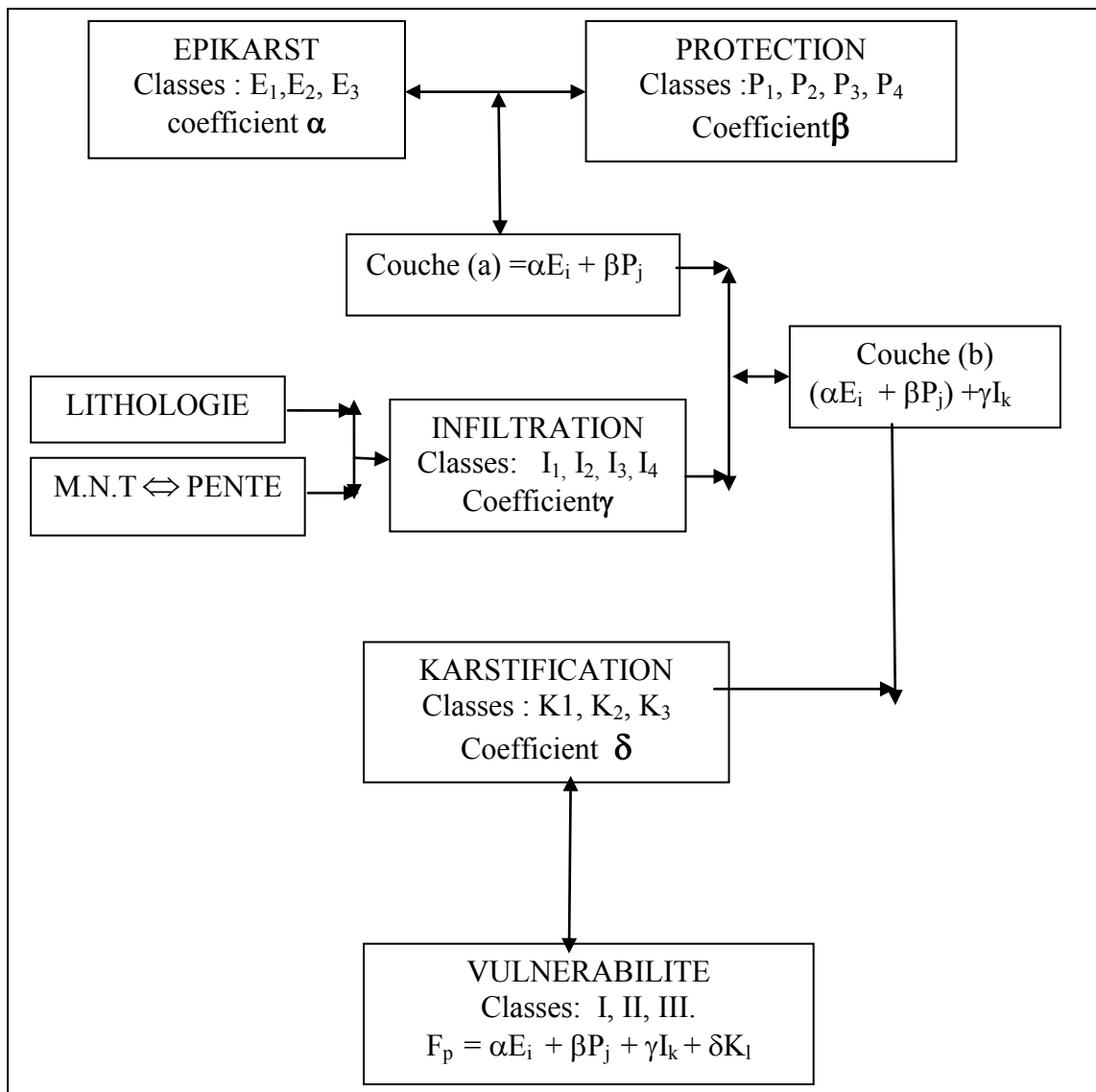
Figure 101: Diagramme des croisements de couches d'information EPIK.
