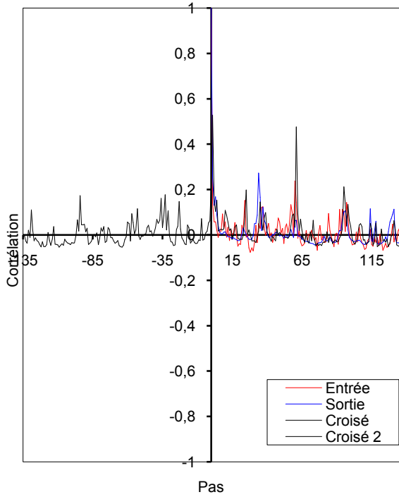
Corrélogrammes simples et croisés Troncature : 135 jours Pas : 1440 min Pas de calcul : 1 PK50-1995-96
