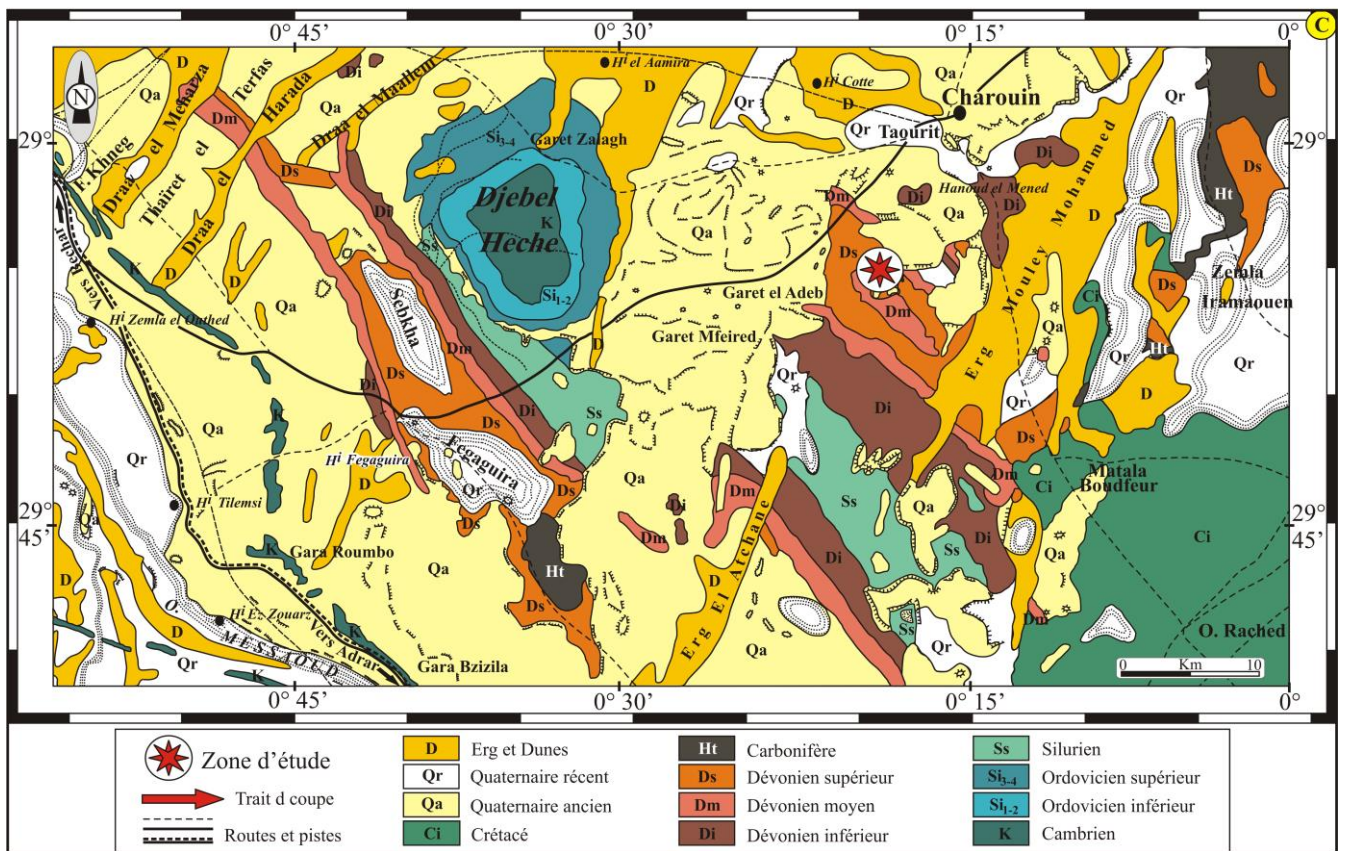
Figure 2 : Cadre géologique des trois régions étudiées : (A) bassin de Béchar (Ben Zireg) (d'après Pareyn, 1961, modifié) ; (B) bassin de l'Ougarta (Marhouma) (image d'arrière-plan d'après Google Earth) ; (C) bassin du Gourara (Charouine) (Carte de Kerzaz, modifiée)
