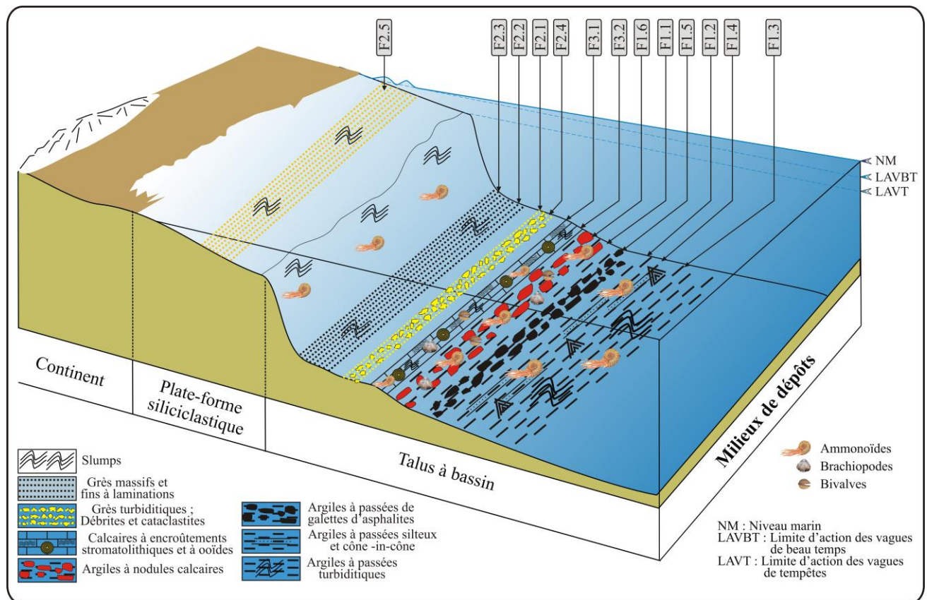
Figure 6 : Bloc diagramme montrant la répartition des faciès et des associations de faciès dans des environnements de plate-forme détritique et de bassin. F1.1 = Argiles noires (« black shales »), F1.2 = Argiles à passées de silts et calcisiltites, F1.3 = Argiles à passées turbiditiques, F1.4 = Argiles à passées de calcaires silteux à « cône-in-cône », F1.5 = Argiles à passées de calcaires à nodules noirs micritiques, F1.6 = Argiles à nodules calcaires, F2.1 = Grès turbiditiques, F2.2 = Grès fins à laminations, F2.3 = Débrites, F2.4 = Grès massifs
