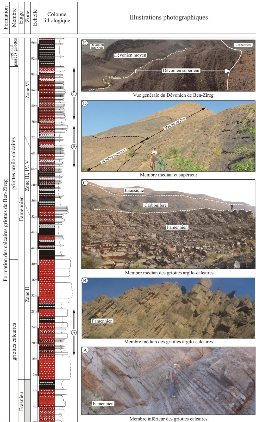
Figure 3 : Succession lithostratigraphique du Dévonien supérieur de Ben-Zireg (bassin de Béchar)
