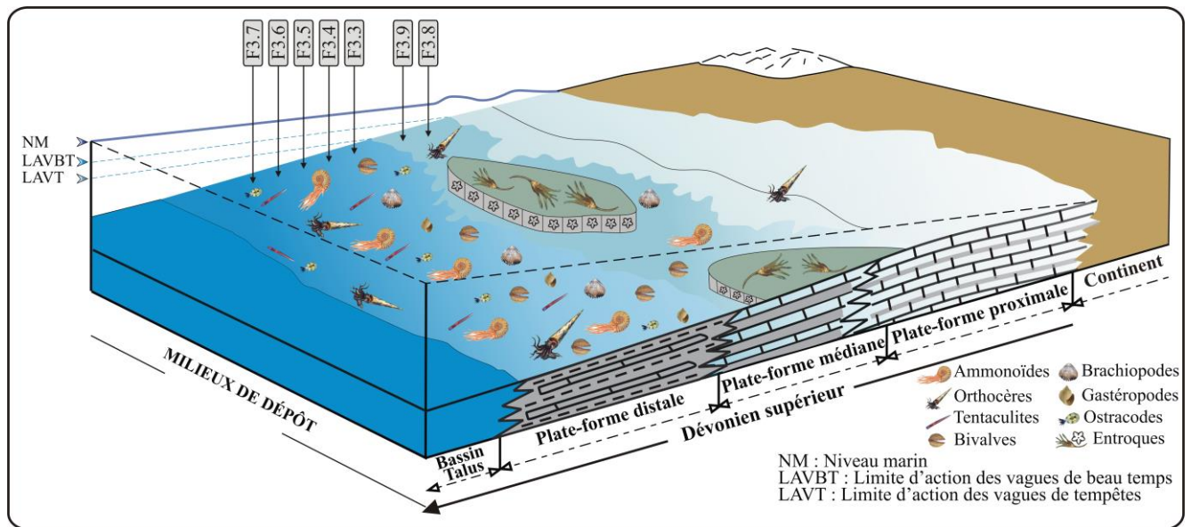
Figure 8 : Modèle schématique de répartition des sous-faciès et des environnements de dépôts des grottes dans une plate-forme carbonatée de type rampe
