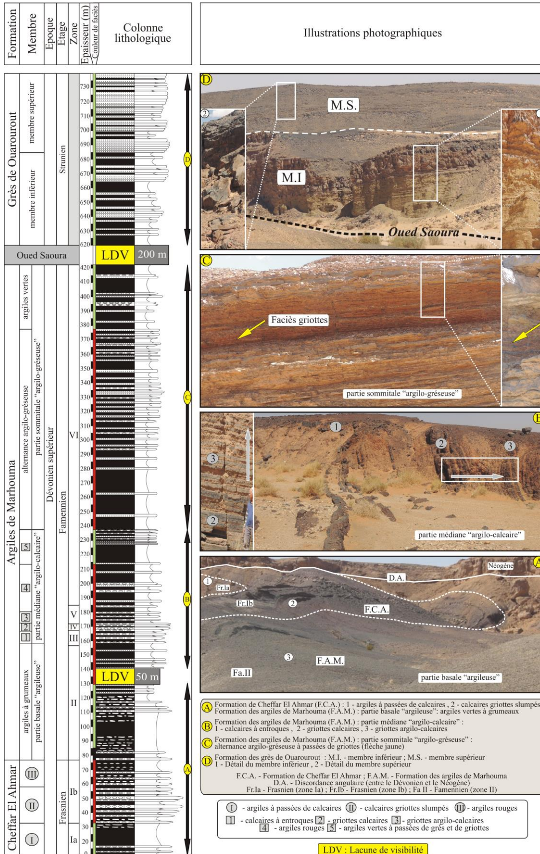
Figure 4 : Succession lithostratigraphique du Dévonien supérieur de Marhouma (bassin de l'Ougarta)
