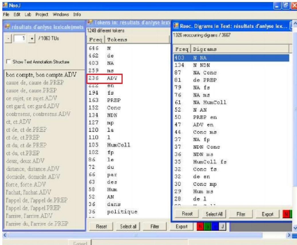
Figure 5 Lemmatisation du corpus avec Nooj
