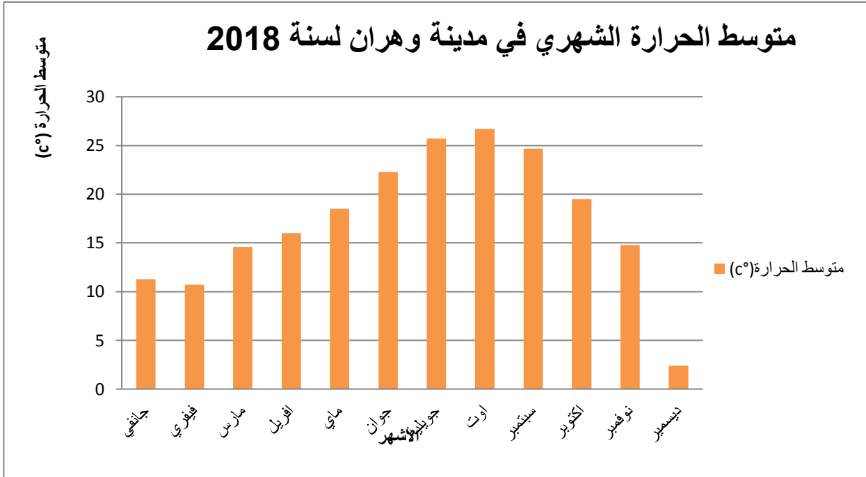
الشكل رقم 01: متوسط الحرارة الشهري بمدينة وهران سنة 2018
