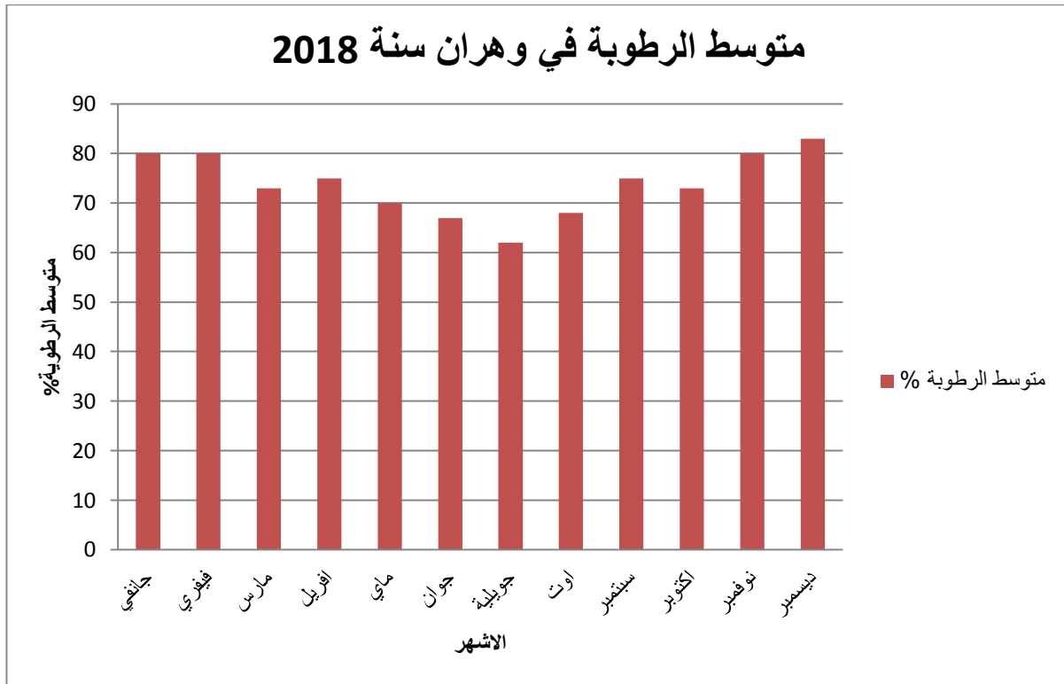
الشكل رقم 03: متوسط الرطوبة في وهران سنة 2018
