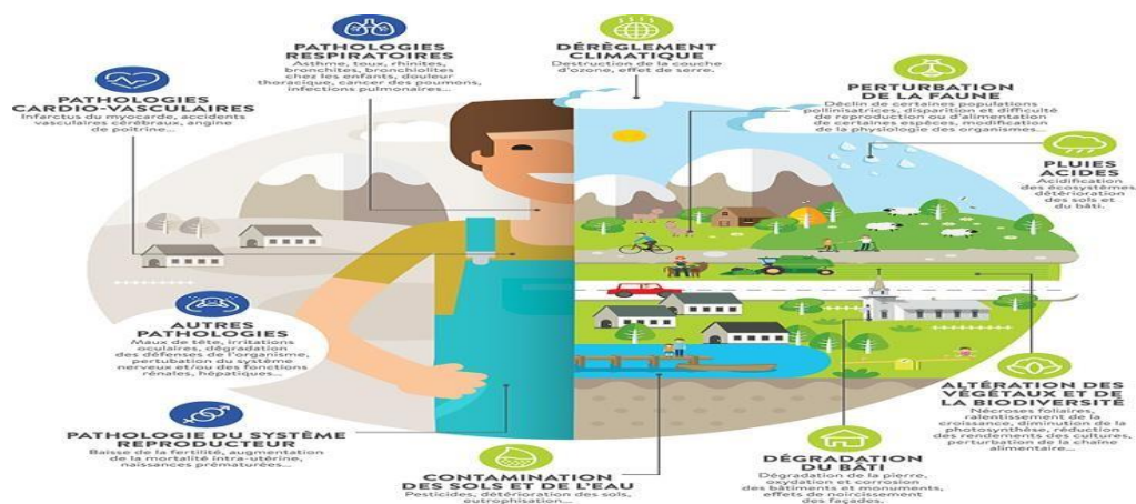
Figure I.3. Effets de la pollution sur l'environnement.
